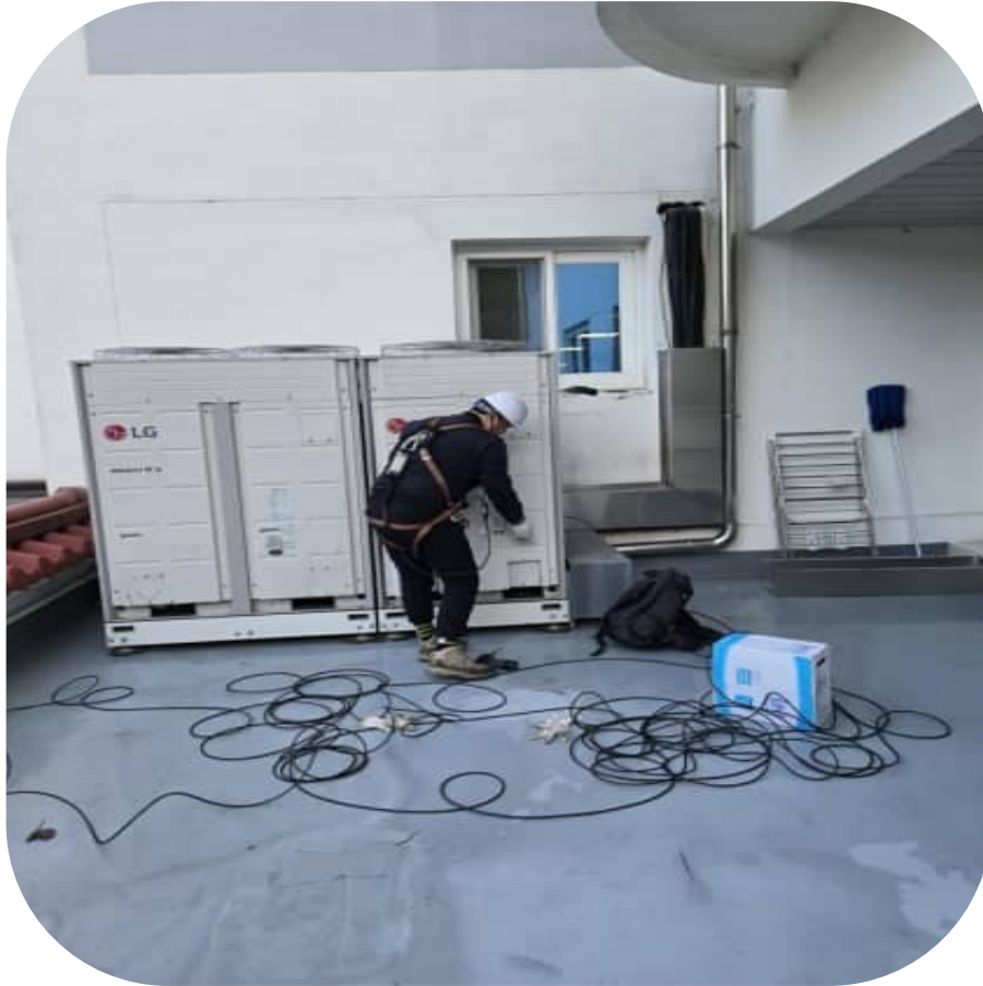
실외기 통신선 작업
