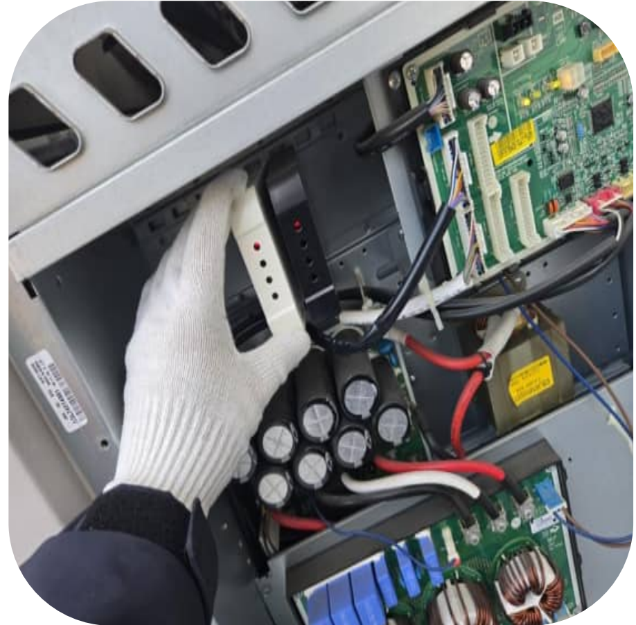
실외기 통신보드 작업
